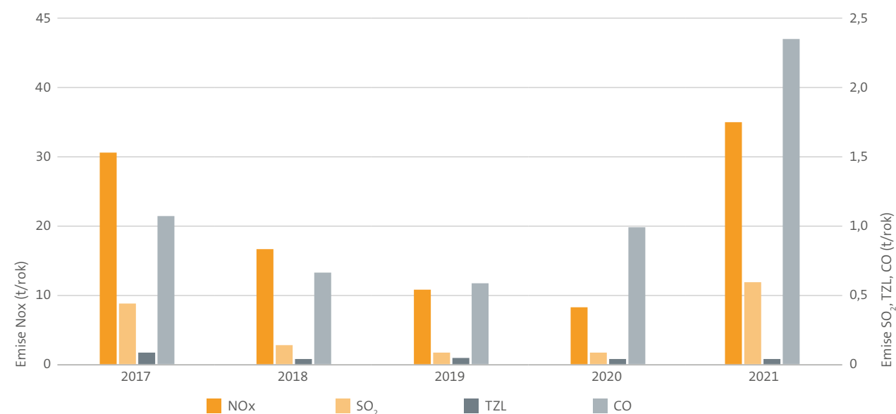
Průběh produkce emisí v Pražské teplárenské za posledních 5 let
