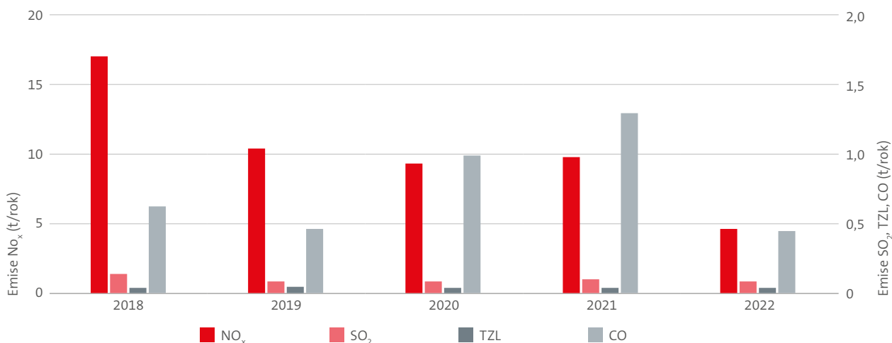
Průběh produkce emisí v Pražské tepleárenské za posledních 5 let
